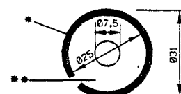
DET H
