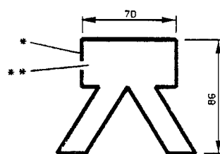
DET G
