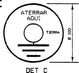
DET C
