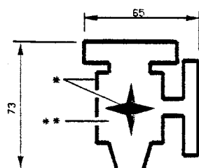
DET D
